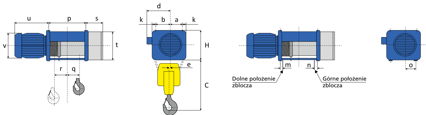
Wciągnik stacjonarny (na łapach) – Seria M, 2 liny (olinowanie 2/1)
